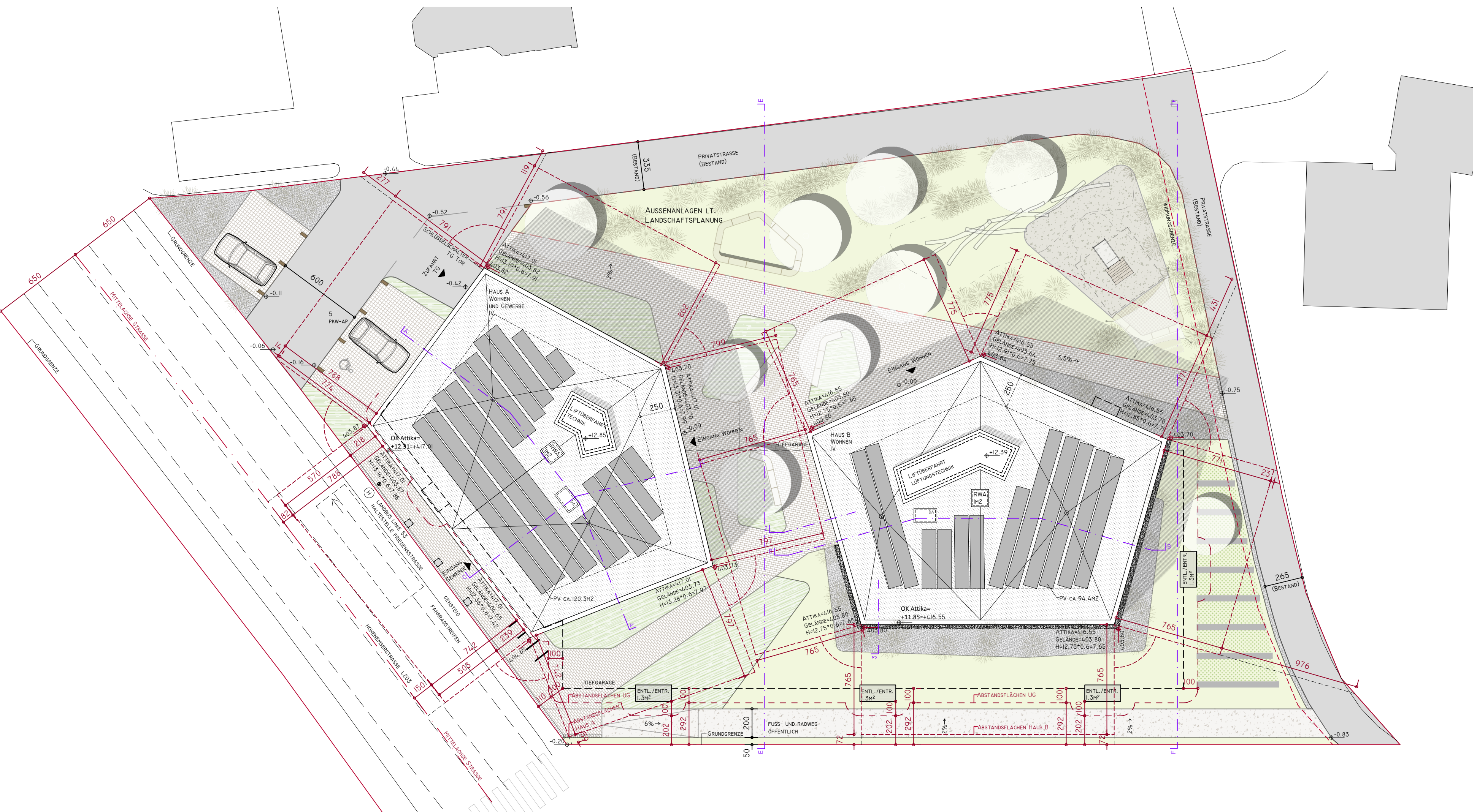
Lageplan M 1:200
